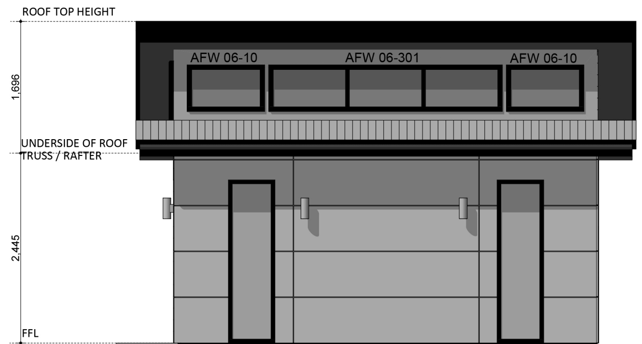
ELEVATION 02
