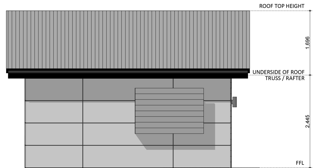
ELEVATION 04
